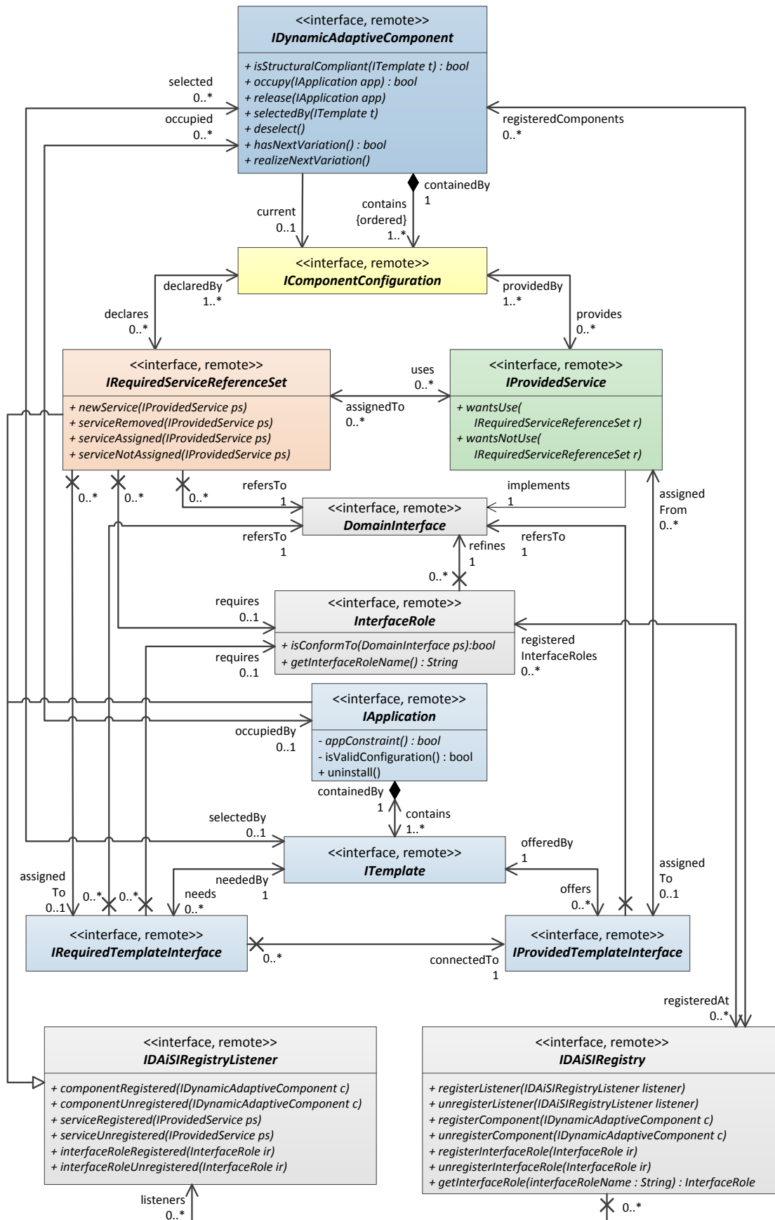
Abbildung 7-1: Die Schnittstellen des Frameworks
