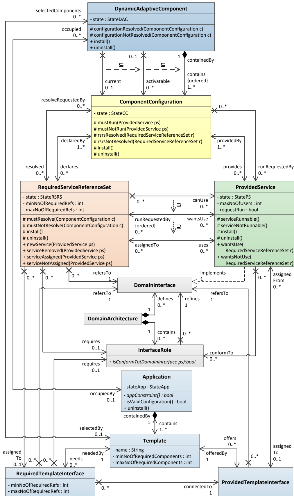
Abbildung 6-8: Das vollständige Komponentenmodell zur Spezifikation und Umsetzung anwendungsglobaler Eigenschaften
