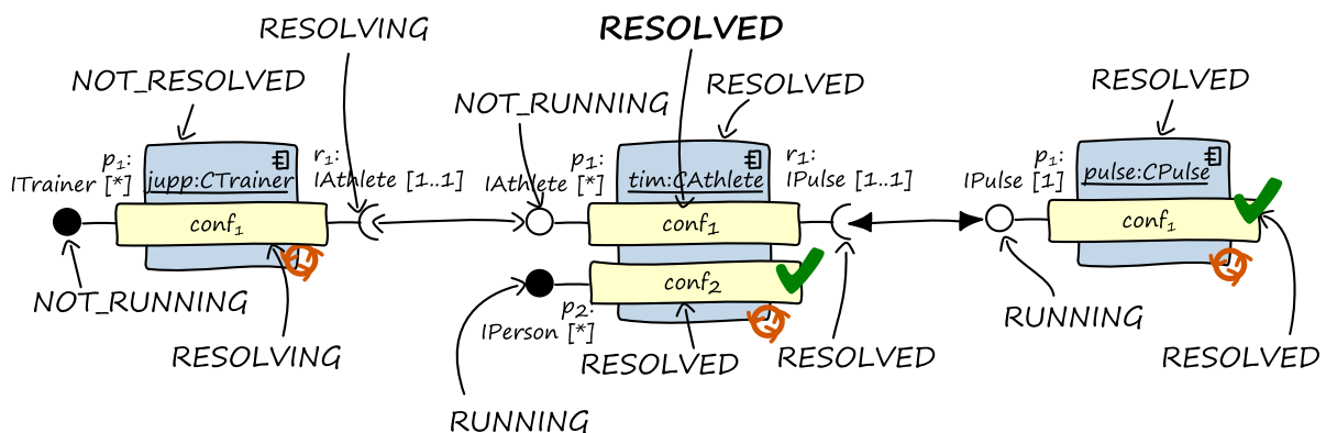
Abbildung 4-37: Die Komponente tim besitzt eine weitere aktivierbare Konfiguration
