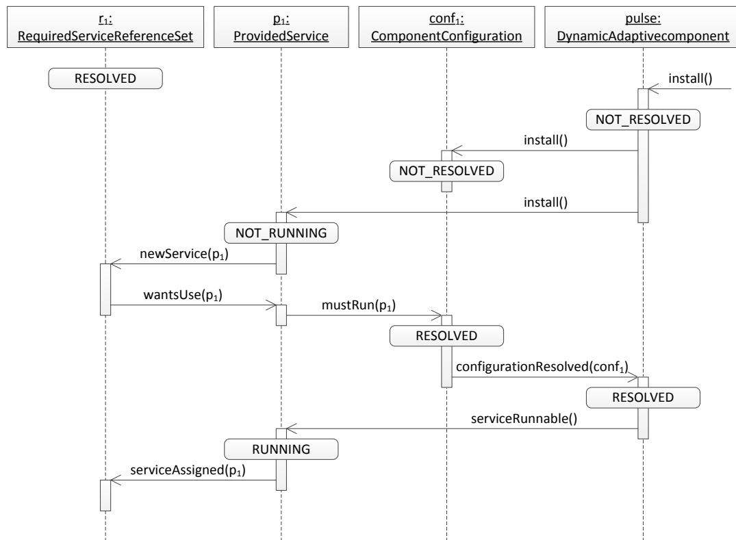
Abbildung 4-21: Komponentenübergreifender Konfigurationsprozess nach Installation der Sportlerkomponente
