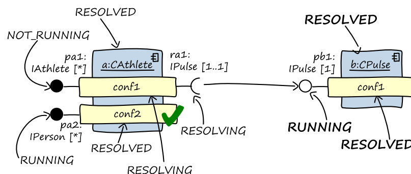
Abbildung 8-15: Situation nach Abschluss des komponenteninternen Konfigurationsprozesses der Pulskomponente
