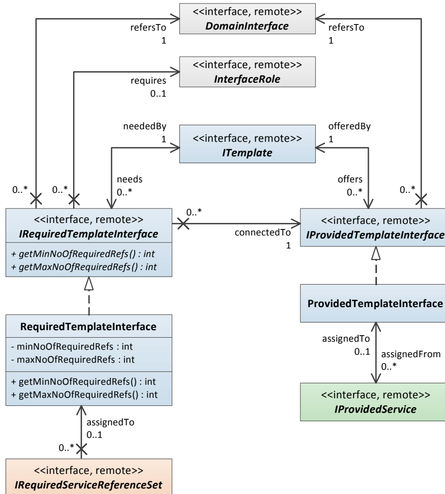
Abbildung 7-9: Realisierung der Klassen ProvidedTemplateInterface und RequiredTemplateInterface des Modells
