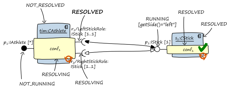
Abbildung 8-11: Zuordnung einer rollenkompatiblen Skistockkomponente
