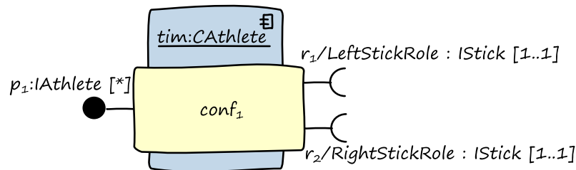
Abbildung 5-3: Athletenkomponente mit zwei RequiredServiceReferenceSets für linken und rechten Skistock
