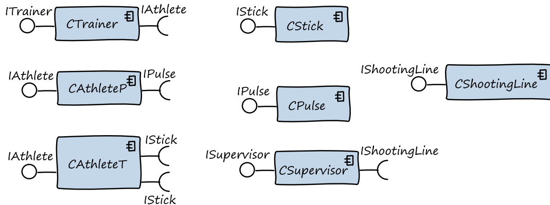
Abbildung 3-2: Die Biathlonkomponenten für das Beispiel
