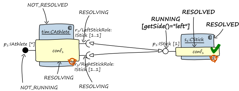
Abbildung 8-10: Die Skistockkomponente kann verwendet werden
