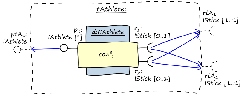
Abbildung 6-14: Beispiel für mögliche Zuordnungen von Komponentenschnittstellen zu Templateschnittstellen
