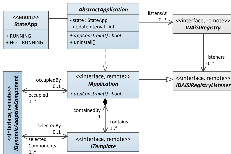
Abbildung 7-7: Realisierung der Klasse Application innerhalb des Frameworks
