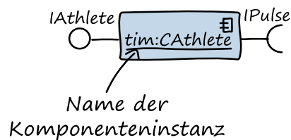
Abbildung 2-2: Beispiel für die grafische Notation einer Komponenteninstanz
