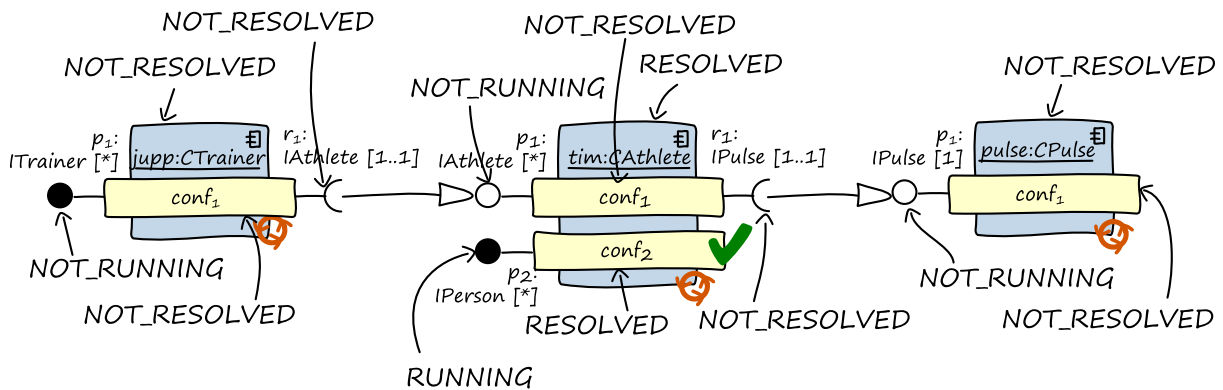
Abbildung 4-28: Eine dritte Komponente wird hinzugefügt
