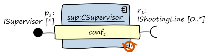
Abbildung 6-4: Die für das System zur Verfügung stehende Schießaufsichtskomponente
