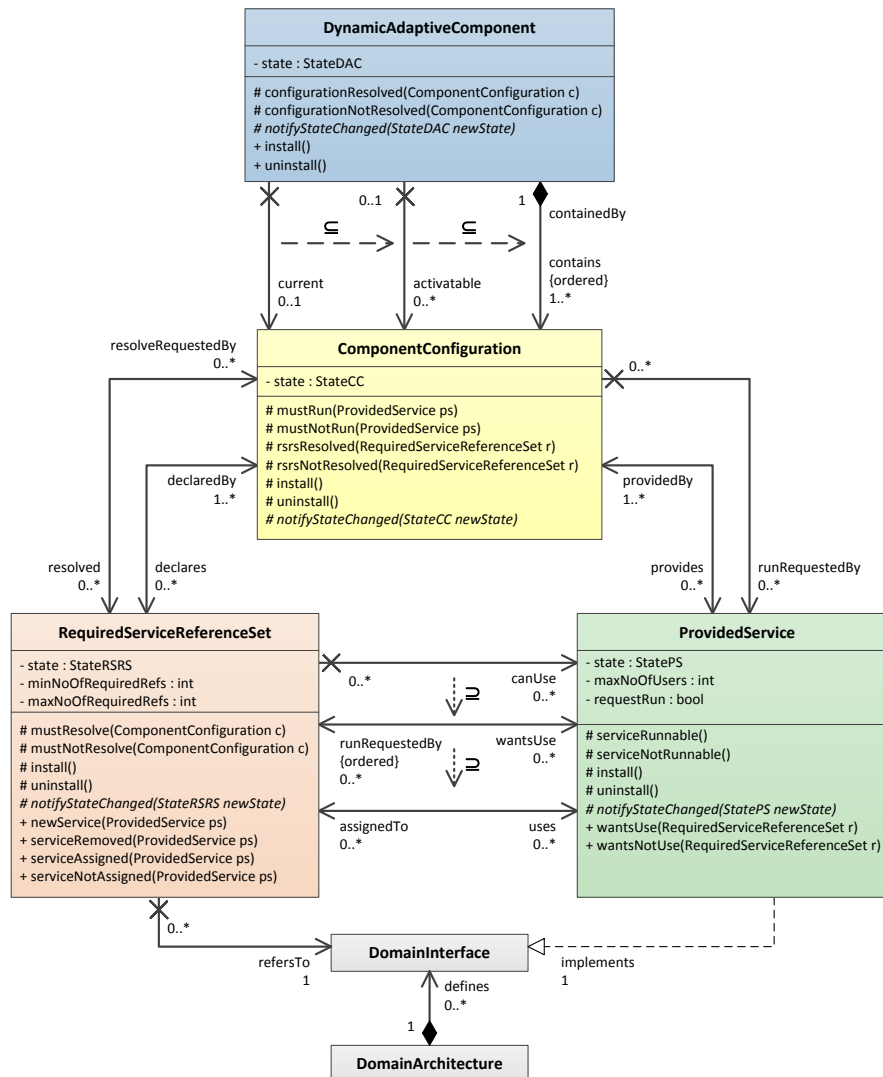
Abbildung 4-5: Komponentenmodell zur Realisierung selbstkonfigurierender Komponenten
