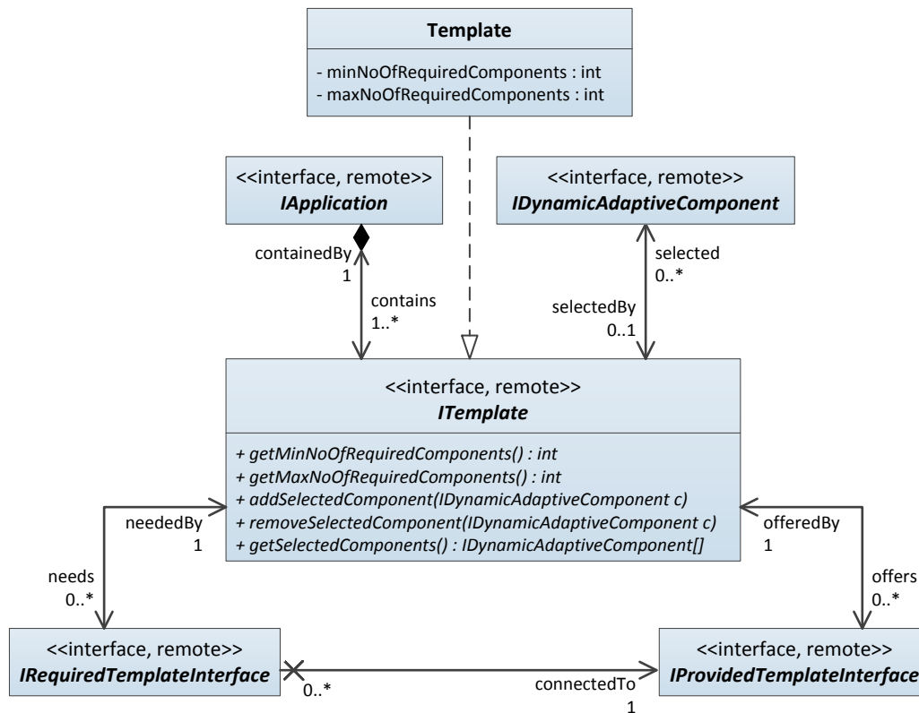
Abbildung 7-8: Die Realisierung der Klasse Template aus dem Modell
