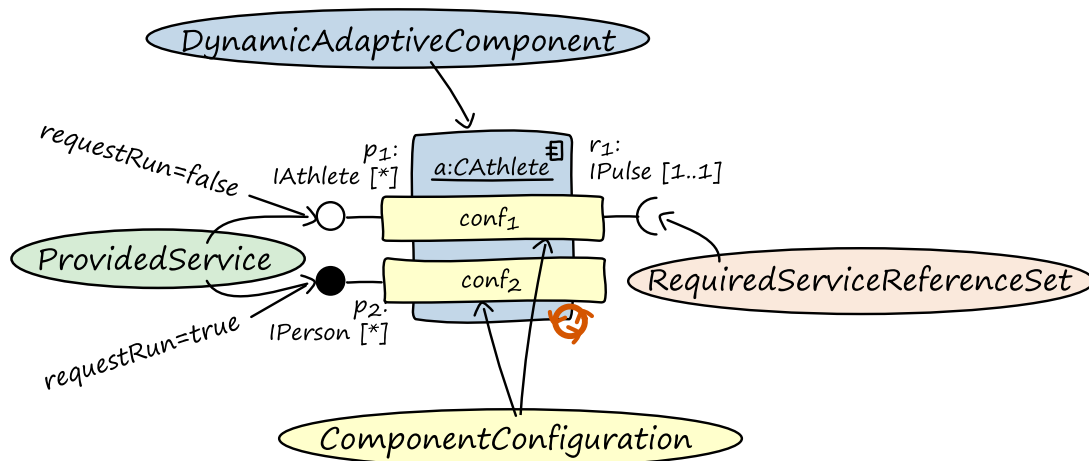
Abbildung 4-6: Beispielnotation einer Komponente
