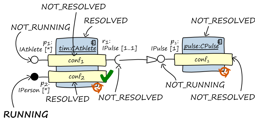
Abbildung 4-27: Das Ergebnis des Konfigurationsprozesses nach Hinzufügen der Athletenkomponente
