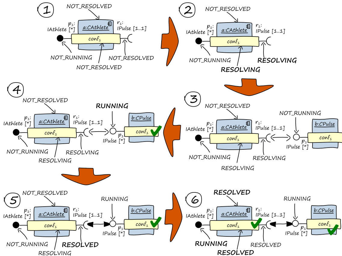
Abbildung 8-5: Beispiel zur Auflösung von Abhängigkeiten
