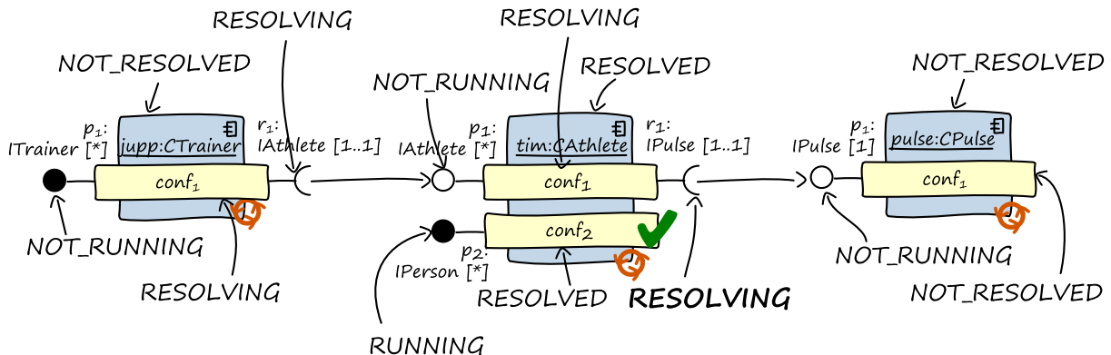
Abbildung 4-32: Das RequiredServiceReferenceSet der Komponente tim wechselt in den Zustand RESOLVING
