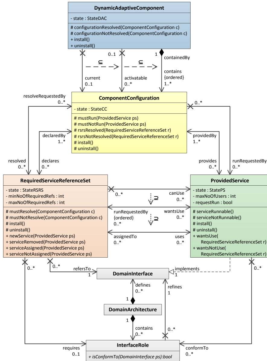
Abbildung 5-2: Erweiterung des Komponentenmodells um Schnittstellenrollen
