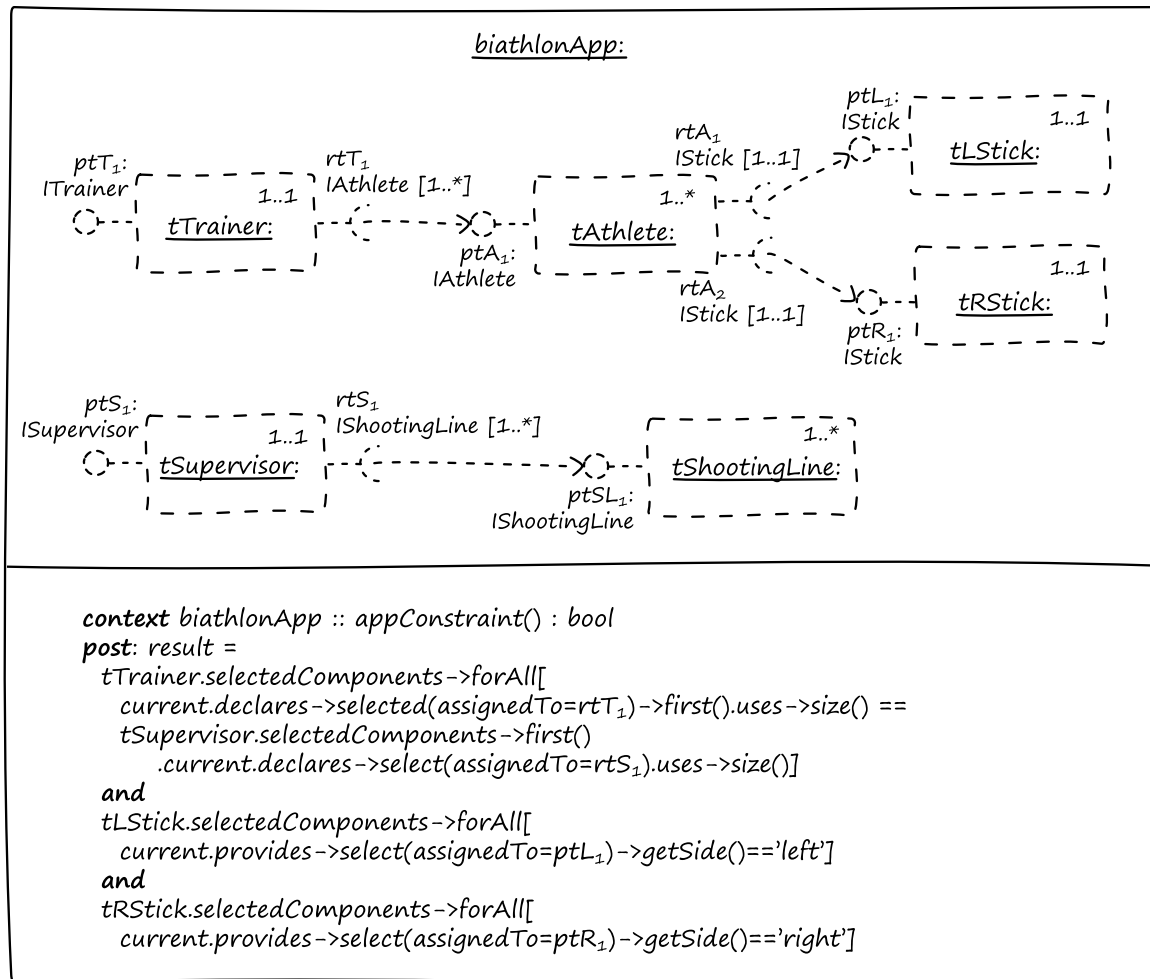
Abbildung 6-9: Beispiel der grafischen Darstellung einer Anwendungsspezifikation
