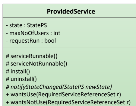
Abbildung 4-12: Die Klasse ProvidedService
