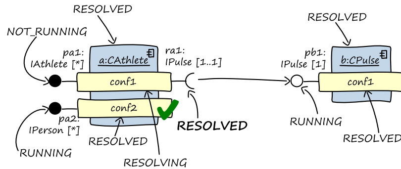
Abbildung 8-16: Die Situation nach Zuweisung des Pulsdienstes an die Athletenkomponente
