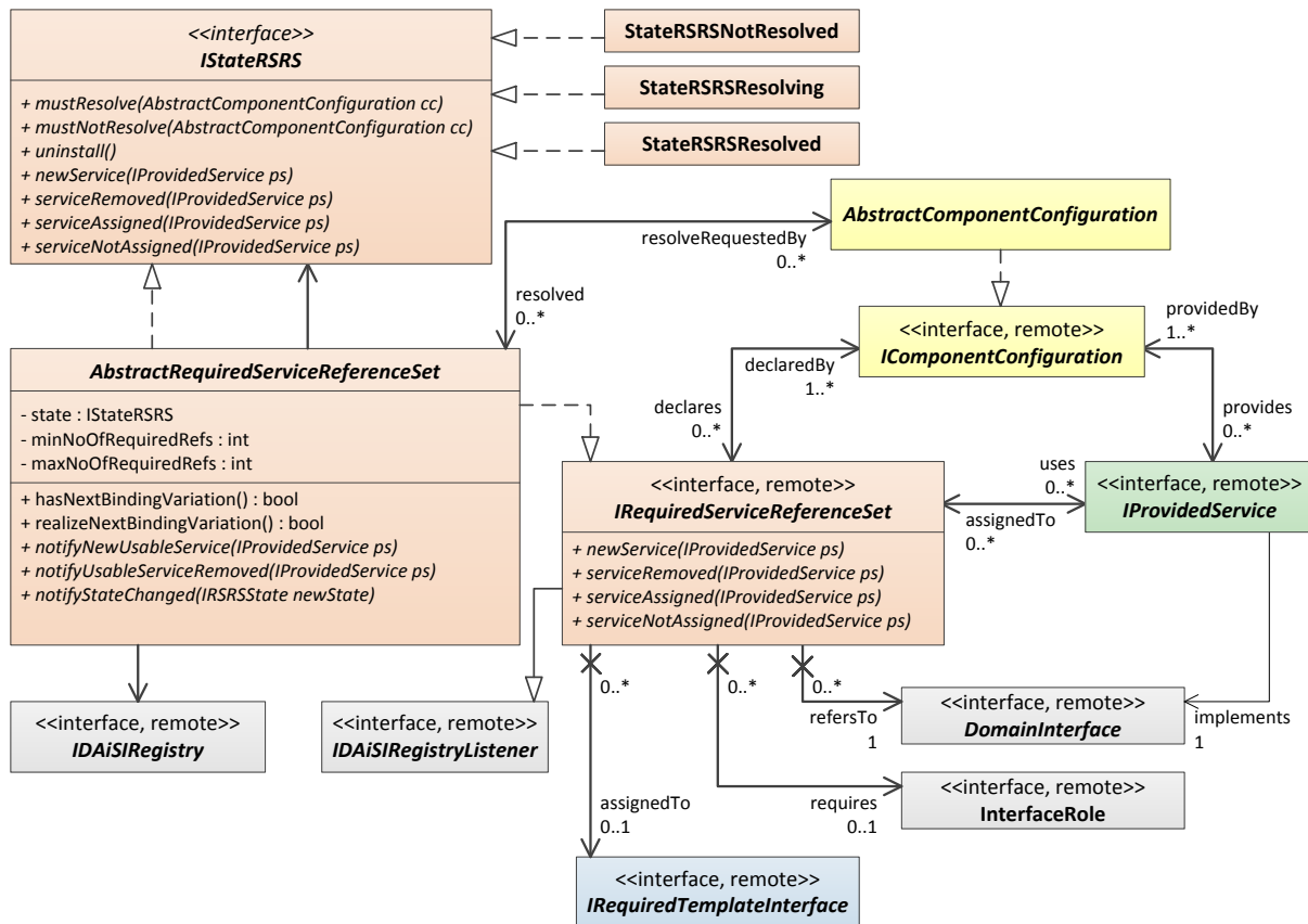
Abbildung 7-6: Realisierung von RequiredServiceReferenceSet des Komponentenmodells
