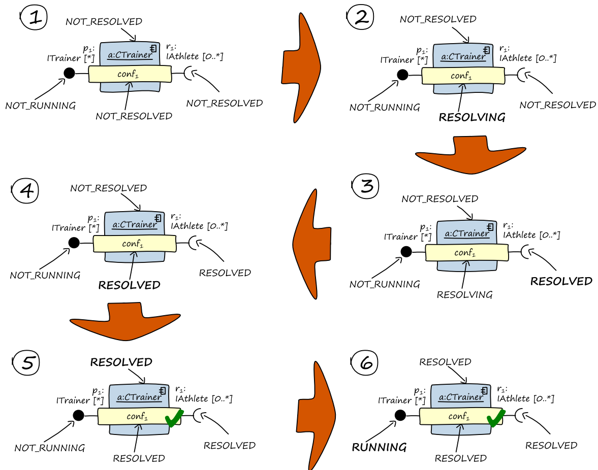
Abbildung 8-2: Beispiel zu gesetztem requestRun -Flag
