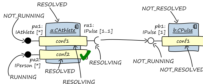
Abbildung 8-14: Situation unmittelbar nach Installation der Pulskomponente
