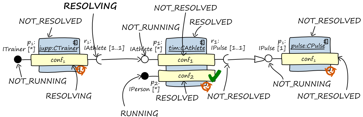
Abbildung 4-30: Das RequiredServiceReferenceSet r_1 der Trainerkomponente wechselt in den Zustand RESOLVING
