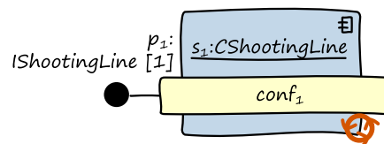
Abbildung 6-3: Die für das System zur Verfügung stehende Schießstandkomponente
