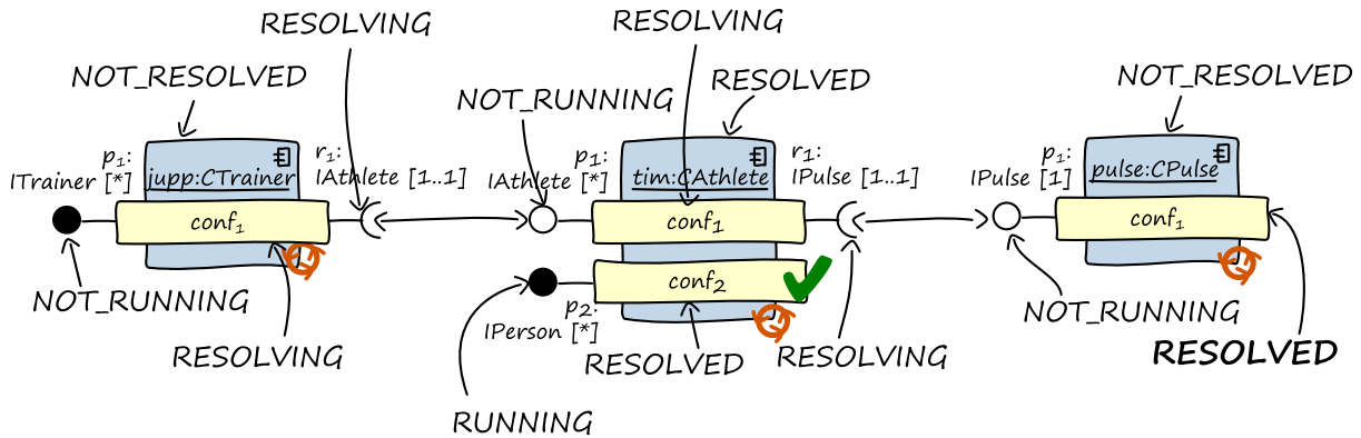
Abbildung 4-33: Die Konfiguration der Pulskomponente wechselt in den Zustand RESOLVED
